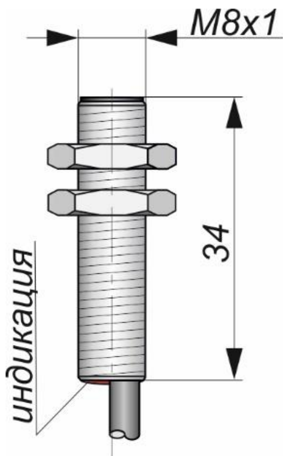
Габаритный чертеж
